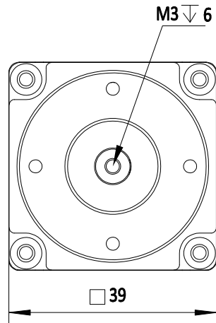
视图 A
