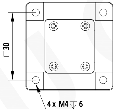
视图 A
