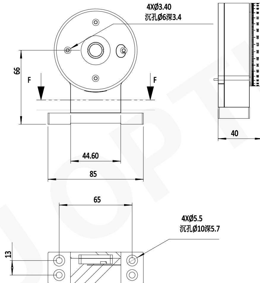
剖面F-F
