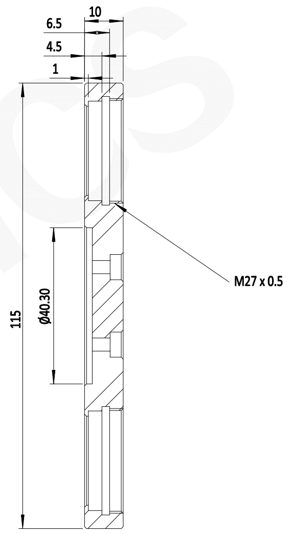
剖面D-D 比例1: 1
