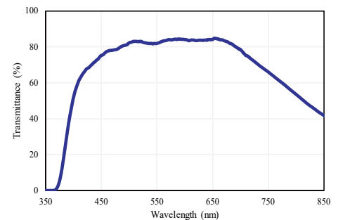
透过率曲线
