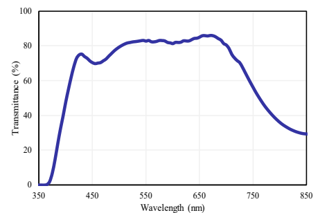
透过率曲线
