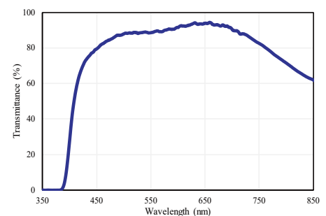
透过率曲线
