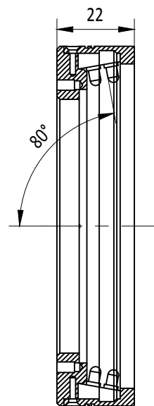
剖视图A-A
