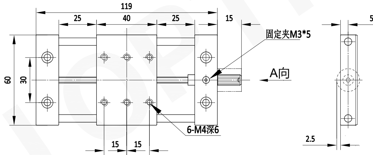
A向视图
